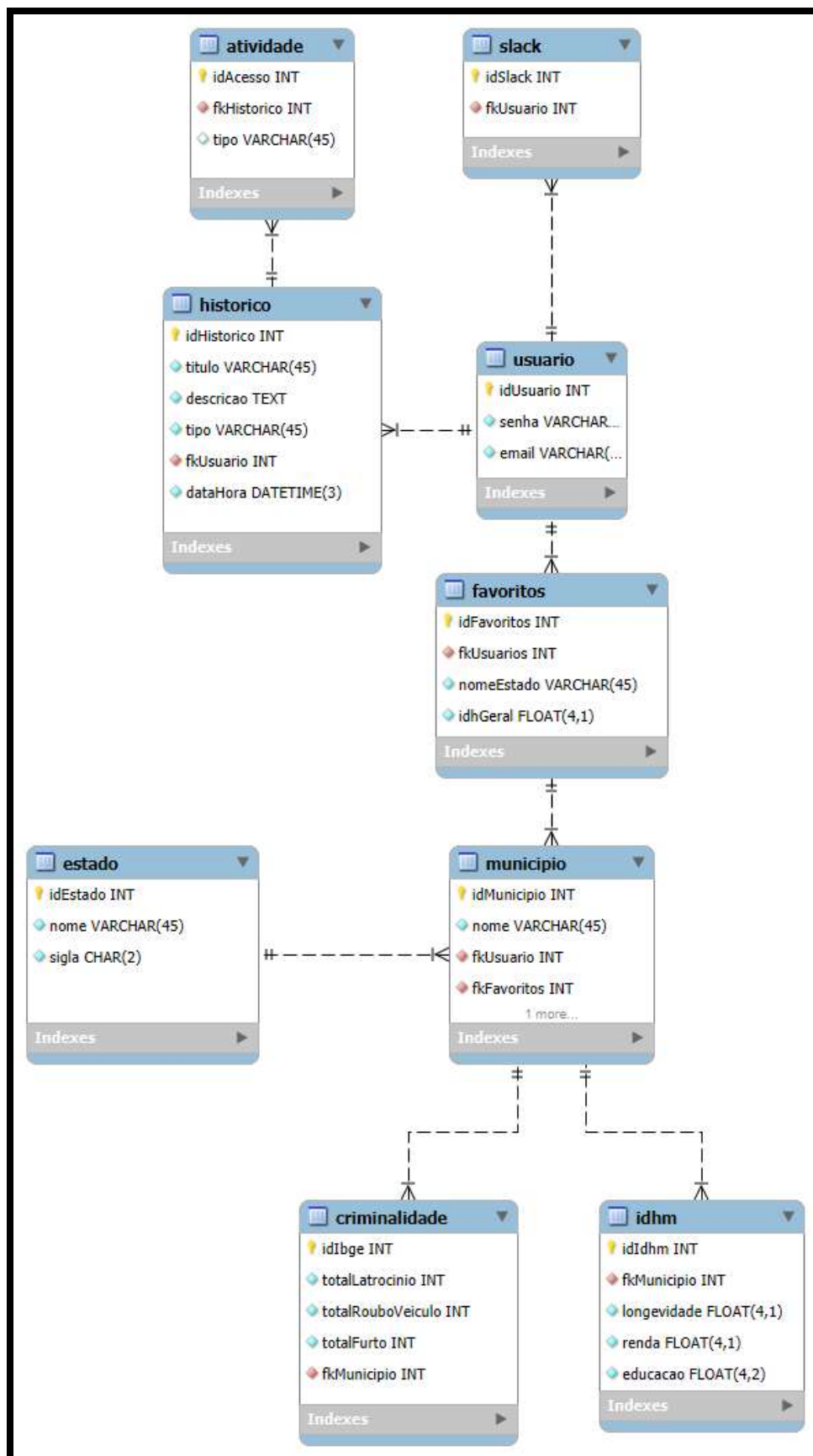
Figura 33 – Diagrama Entidade-Relacionamento (DER).
