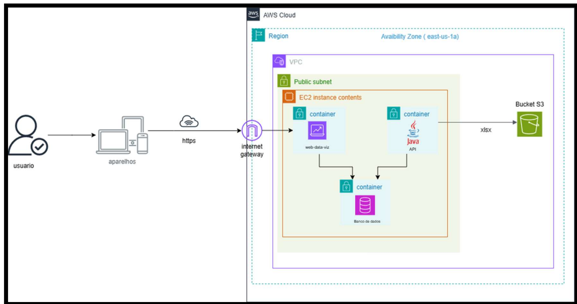
Figura 31 – Arquitetura da Solução.
